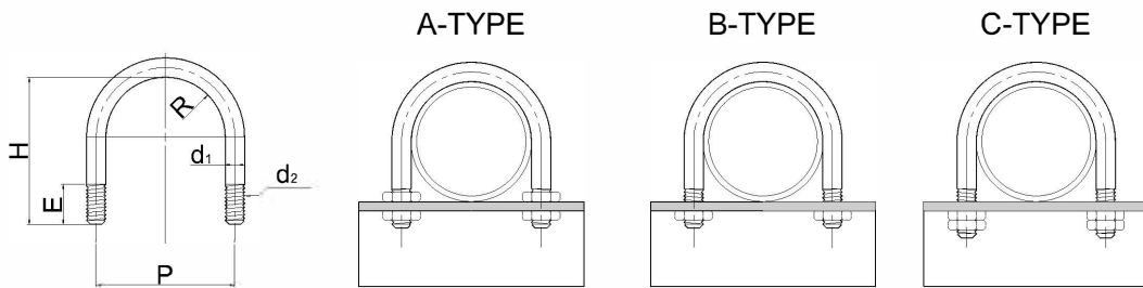
U-BOLT (KS V3032, JIS F3022)
